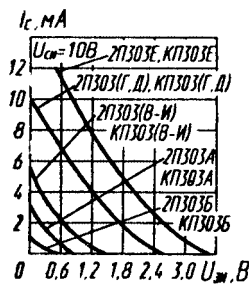
Проходные характеристики
